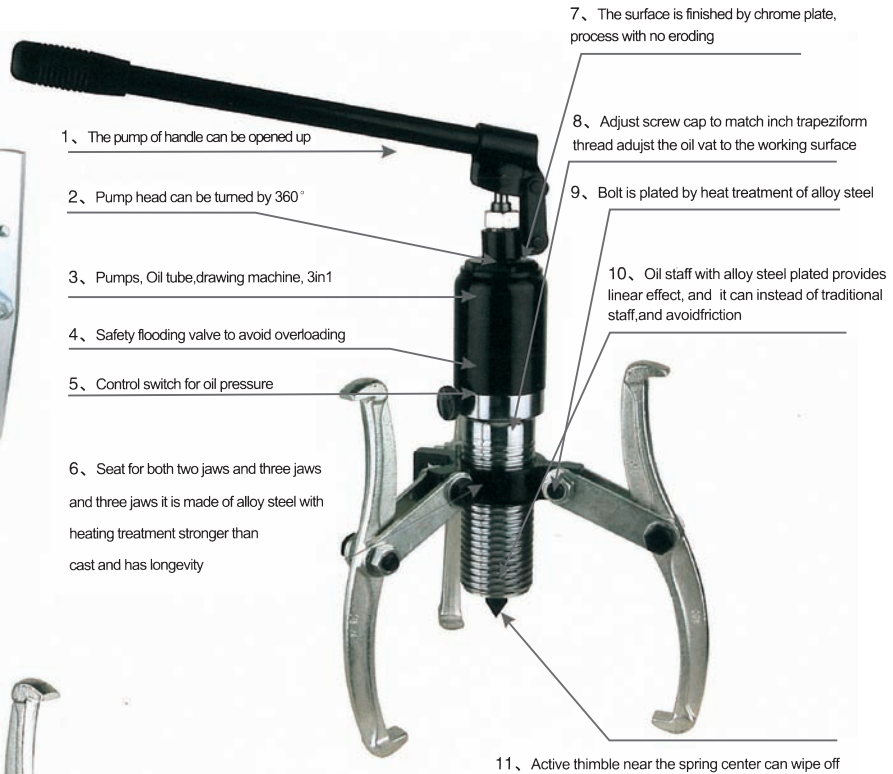
Item No: CK Integral-unit style
